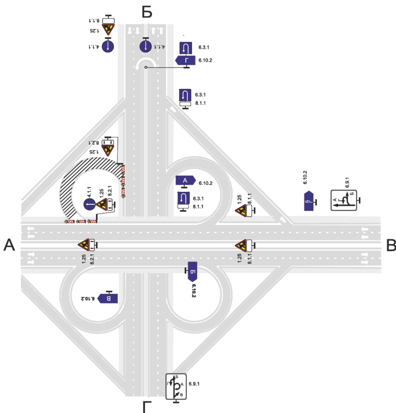
Рисунок Б.31 - Транспортная развязка - клеверный лист. Зона производства работ на левоповоротном съезде. Пропуск транспортных средств по правоповоротному съезду с устройством разворота на одной из дорог
