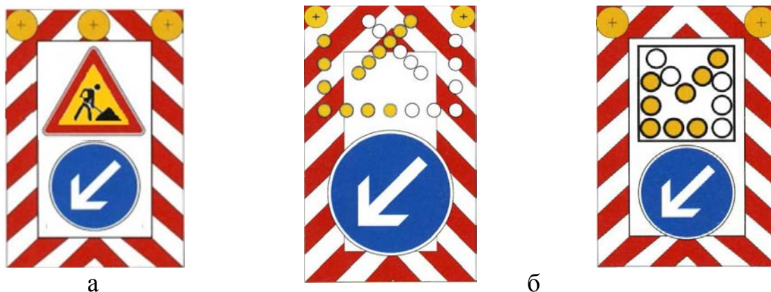
Рисунок 13 – Примеры передвижных заградительных знаков со световой индикацией: а – без мигающей стрелы; б – с мигающей стрелой
